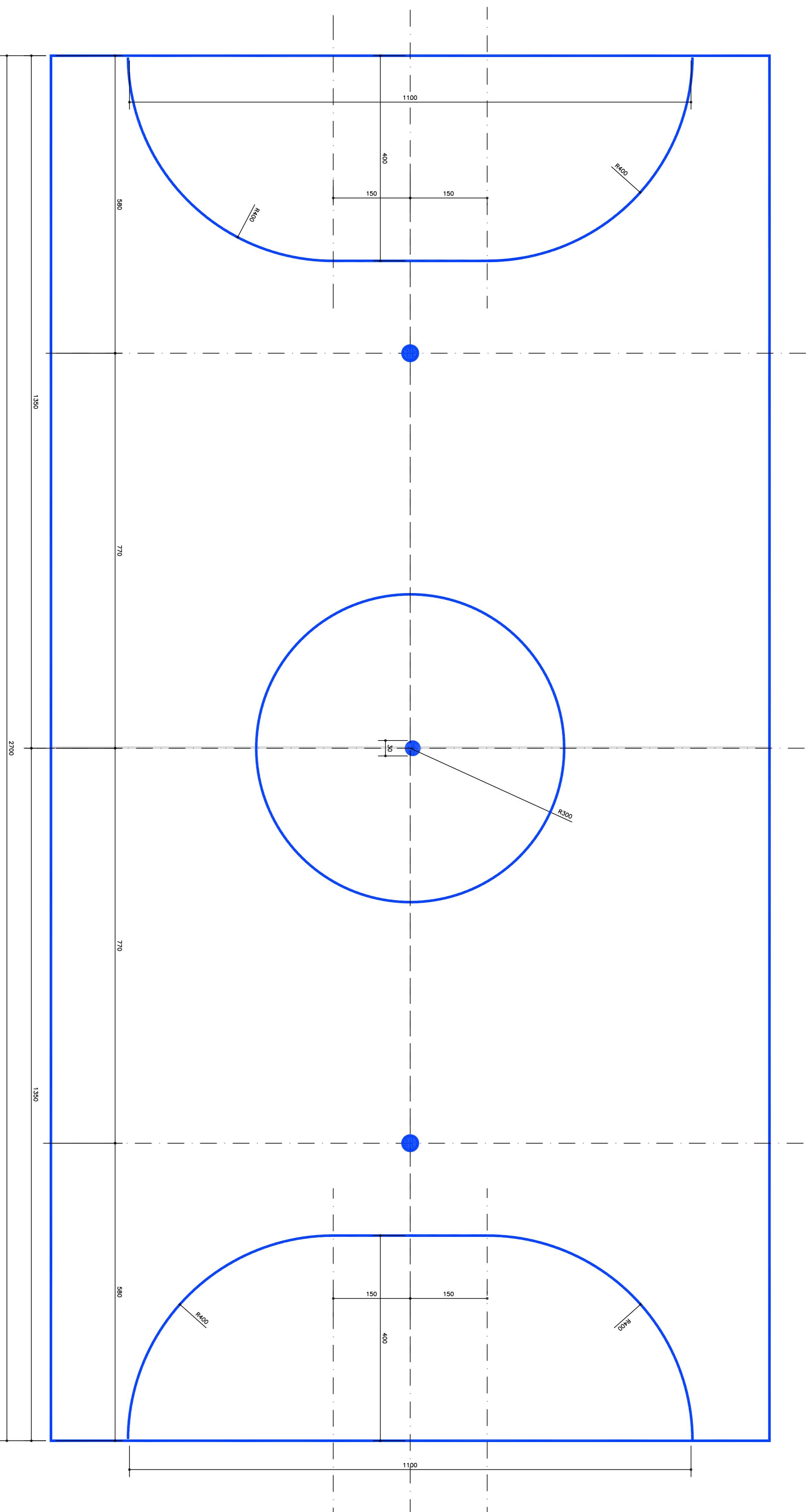
DEMARCAÇÃO DA QUADRA DE FUTEBOL DE SALÃO Folha 07 de 08 (Quadra com 2700) (Arquiteta da Fava Preta - 5cm) ESCALA: 1:50
